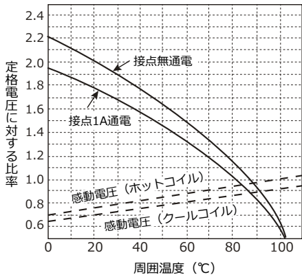
周囲温度—最大印加電圧・感動電圧特性 (18VDCコイル)
