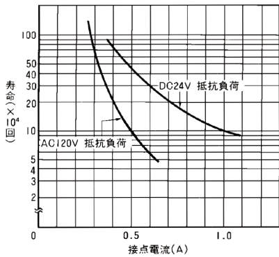
寿命曲線
