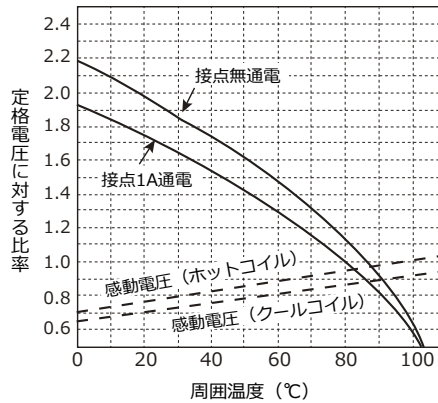
周囲温度—最大印加電圧・感動電圧特性 (24VDCコイル)
