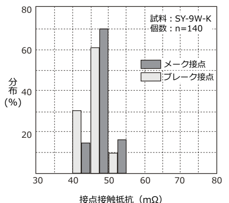
接点接触抵抗の分布
