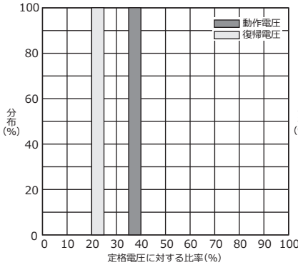
動作・復帰電圧の分布 (2.0 A タイプ)
