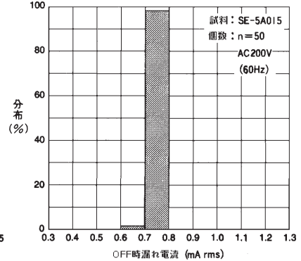
OFF 時漏れ電流の分布
