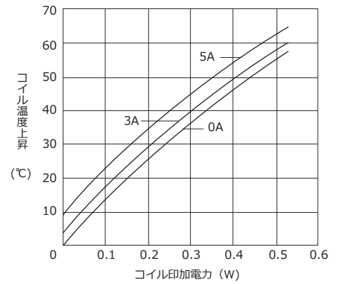
コイル温度上昇特性
