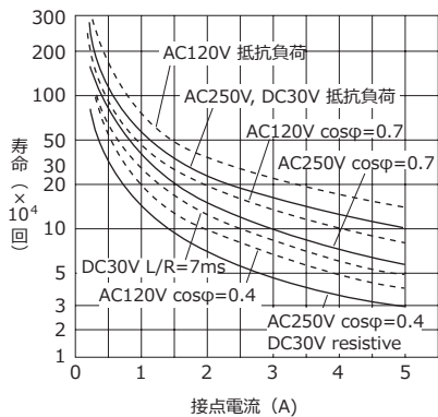
寿命曲線
