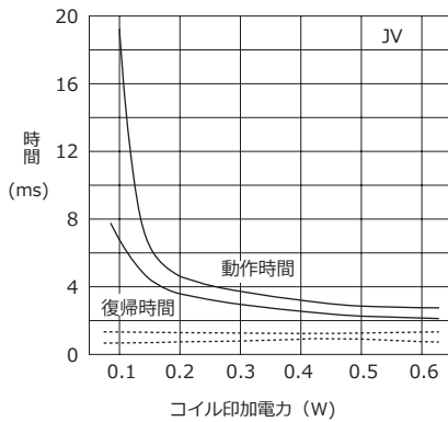
動作・復帰時間特性
