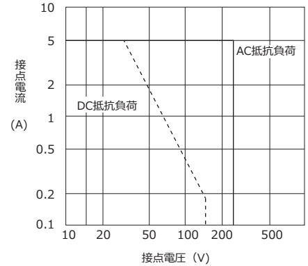
開閉容量の最大値
