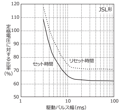
パルス動作特性
