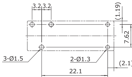
●基板孔開け図 (JSL形) (BOTTOM VIEW)
