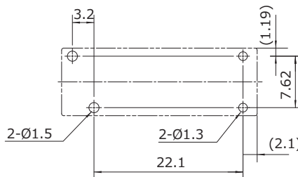
●基板孔開け図 (JSL-M形) (BOTTOM VIEW)
