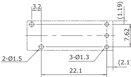
●基板孔開け図 (JSL-DM形) (BOTTOM VIEW)
