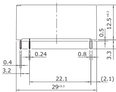
●外形寸法図 (JSL-DM形)
