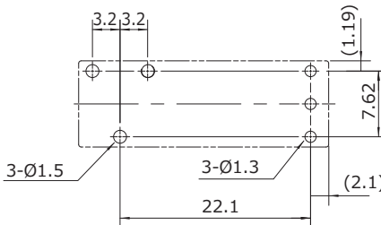
●基板孔開け図 (JSL-D形) (BOTTOM VIEW)
