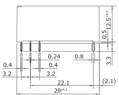
●外形寸法図 (JSL-D形)
