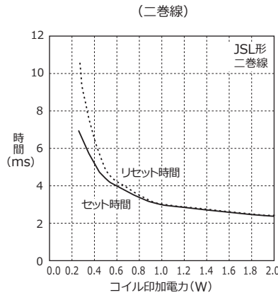
セット・リセット時間特性
