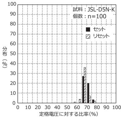
セット・リセット電圧の分布
