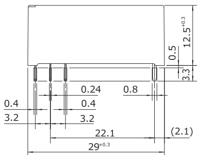
●外形寸法図 (JSL形)
