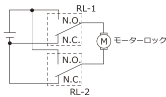
・試験回路
