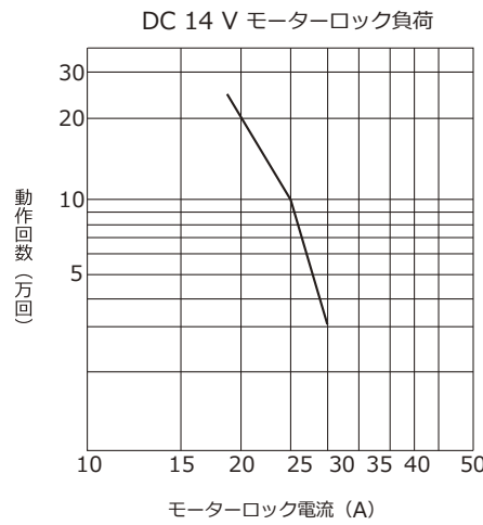
寿命曲線
