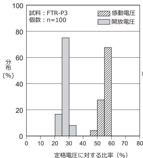
感動・開放電圧の分布
