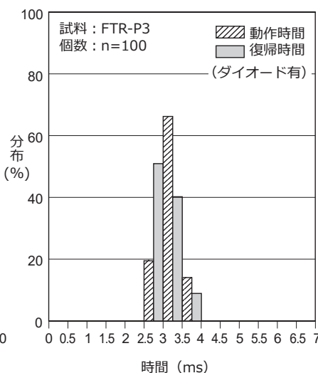
動作・復帰時間の分布
