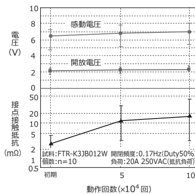
電氣的寿命試験 (抵抗負荷) (感動・開放電圧、接触抵抗)
