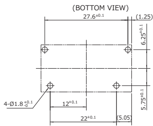
●基板孔開け図 (FTR-K3AB形、FTR-K3JB形)
