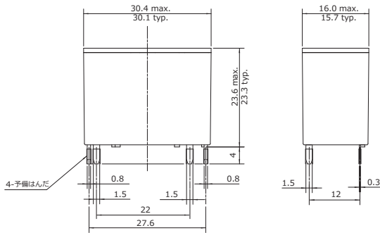
●外形寸法図 (FTR-K3AB形)
