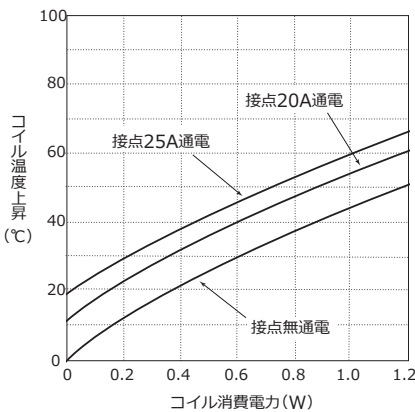
コイル温度上昇特性
