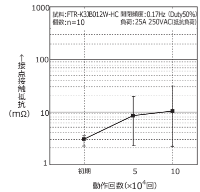
(接触抵抗)
