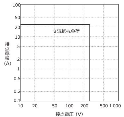
開閉容量の最大値 (電氣的寿命を保証するものではありません)
