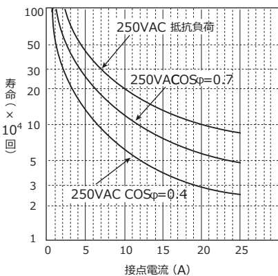
寿命曲線
