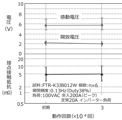
電氣的寿命試験 (インバーター負荷) (感動・開放電圧、接触抵抗)
