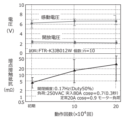
電氣的寿命試験 (モーター負荷) (感動・開放電圧、接触抵抗)
