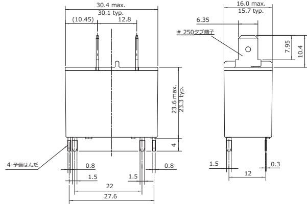
●外形寸法図 (FTR-K3JB形)
