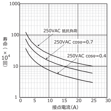
寿命曲線
