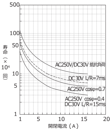
寿命曲線
