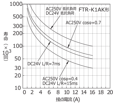
寿命曲線
