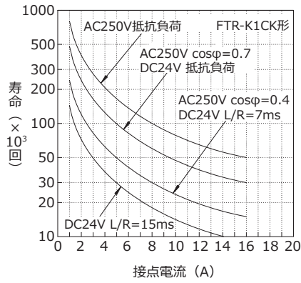
寿命曲線 (1c)
