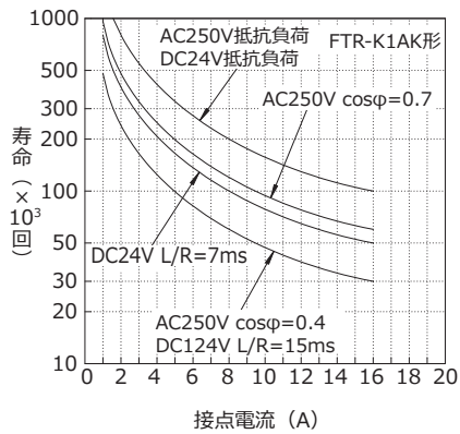
寿命曲線 (1a)
