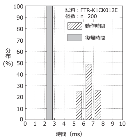
動作・復帰時間の分布
