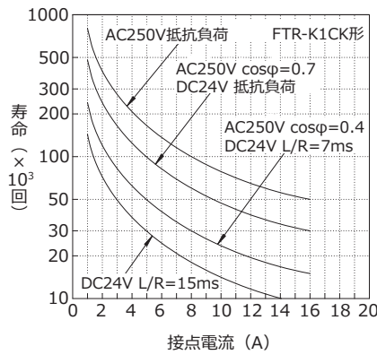
寿命曲線 (1c)
