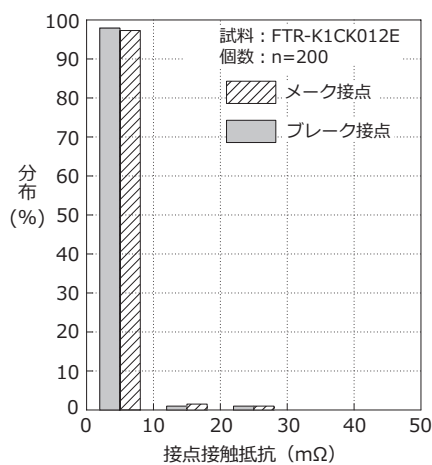
接点接触抵抗の分布
