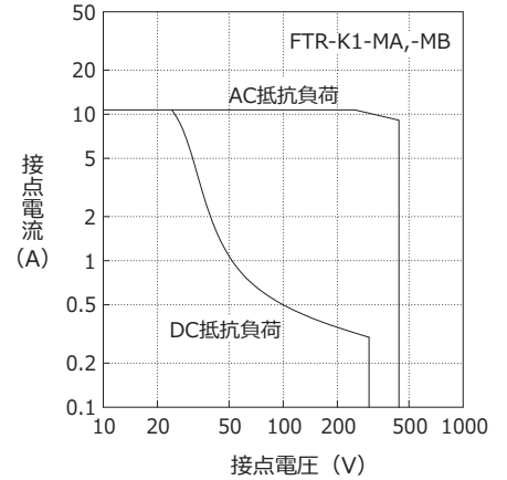
開閉容量の最大値 (電気的寿命を満足するものではありません)
