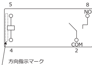
●端子配列・内部結線図 (FTR-K1AK□W-MA) (BOTTOM VIEW)
