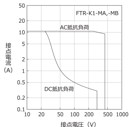
開閉容量の最大値 (電気的寿命を満足するものではありません)
