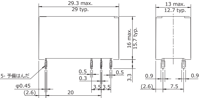
●外形寸法図 (FTR-K1CK□W-MA)
