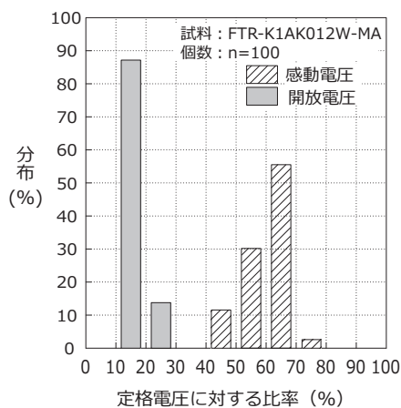
感動・開放電圧の分布
