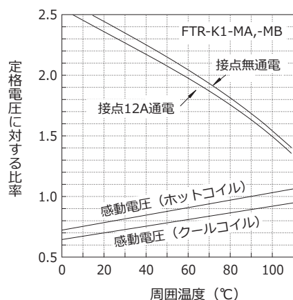
周囲温度—最大印加電圧・感動電圧特性
