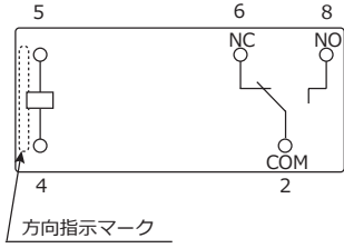
●基板孔開け図 (FTR-K1CK□W-MA) (BOTTOM VIEW)
