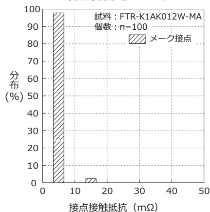
接点接触抵抗の分布
