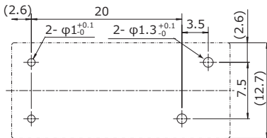
●基板孔開け図 (FTR-K1AK□W-MA) (BOTTOM VIEW)
