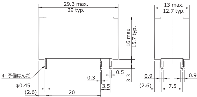
●外形寸法図 (FTR-K1AK□W-MA)
