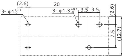
●基板孔開け図 (FTR-K1CK□W-MA) (BOTTOM VIEW)
