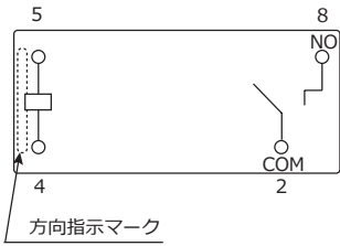
●端子配列・内部結線図 (FTR-K1AK□W-MA) (BOTTOM VIEW)
