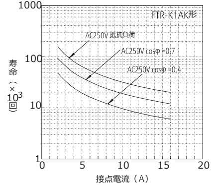
寿命曲線(プラスチックシール形)
