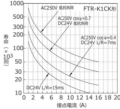
寿命曲線(フラックスフリー形)
