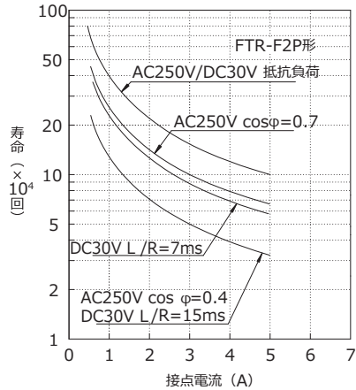
寿命曲線
