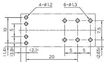
●基板孔開け図 (FTR-F1LDC形) (BOTTOM VIEW)
