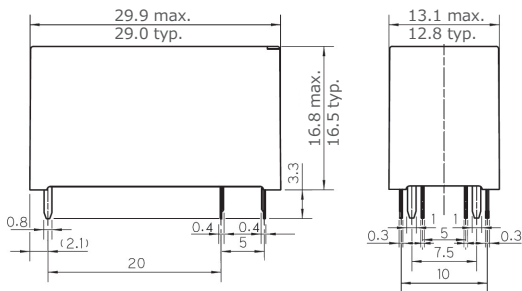
●外形寸法図 (FTR-F1LDA形)
