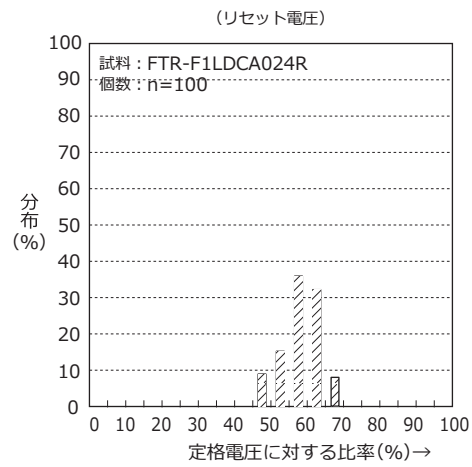
セット・リセット電圧の分布
