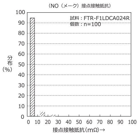
接点接触抵抗の分布
