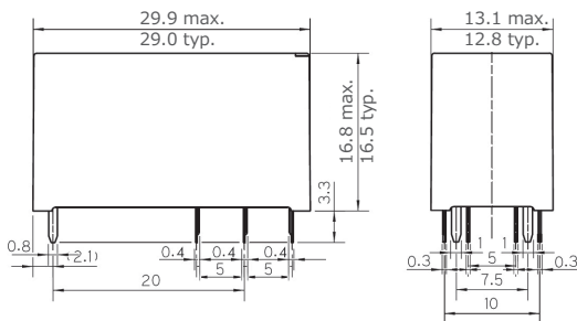
●外形寸法図 (FTR-F1LDC形)
