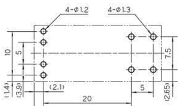
●基板孔開け図 (FTR-F1LDA形) (BOTTOM VIEW)
