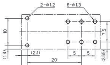
●基板孔開け図 (FTR-F1LC形) (BOTTOM VIEW)
