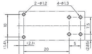
●基板孔開け図 (FTR-F1LA形) (BOTTOM VIEW)
