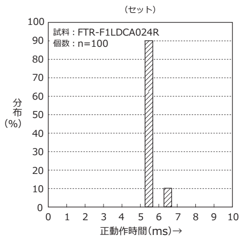
セット・リセット時間の分布
