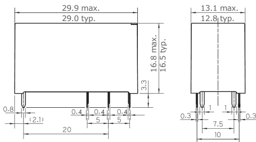
●外形寸法図 (FTR-F1LC形)
