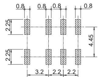
●実装パッド図 (TOP VIEW)
