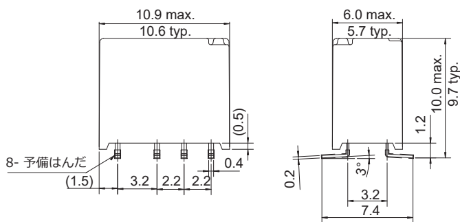
●外形寸法図
