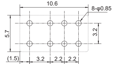
●基板孔開け図 (BOTTOM VIEW)
