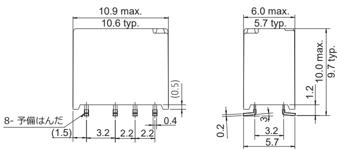
●外形寸法図
