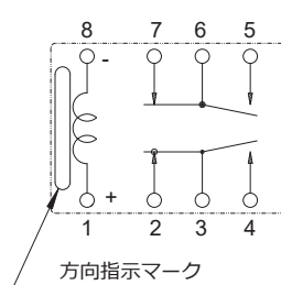
●端子配列・内部結線図 (TOP VIEW)
