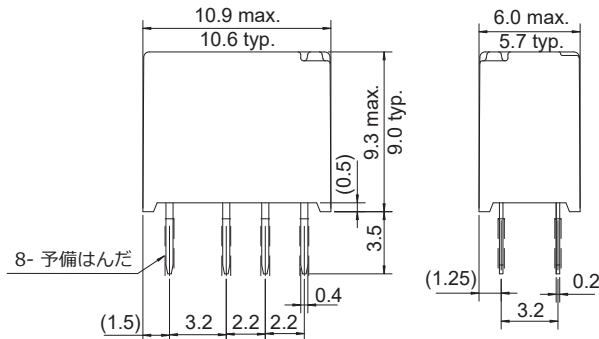
●外形寸法図
