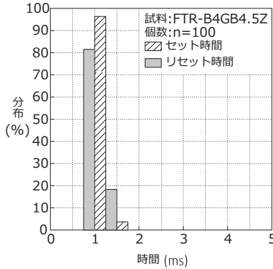
セット・リセット時間の分布
