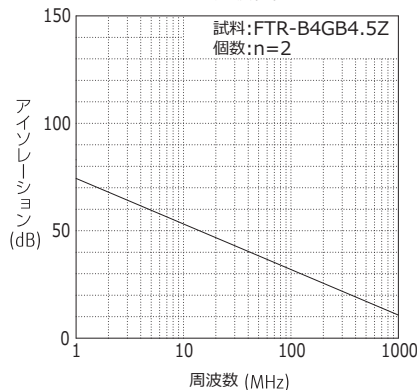
高周波特性
