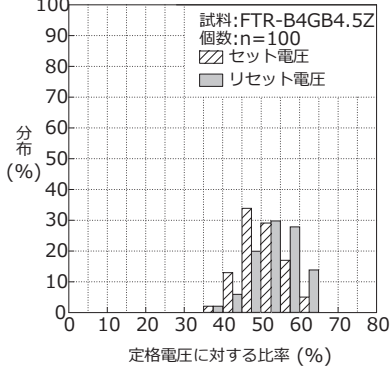
セット電圧・リセット電圧の分布
