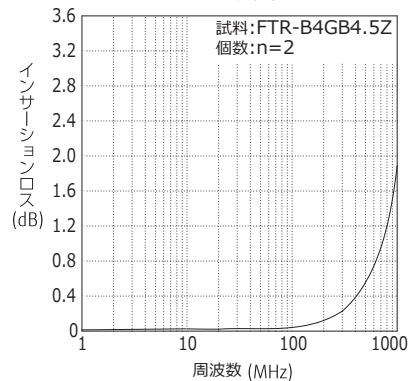
高周波特性
