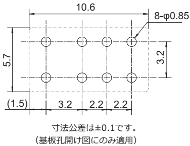
●基板孔開け図 (BOTTOM VIEW)
