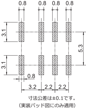
●実装パッド図 (TOP VIEW)
