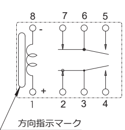
●端子配列・内部結線図 (TOP VIEW)
