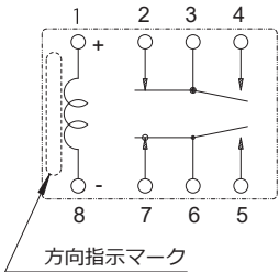
●端子配列・内部結線図 (BOTTOM VIEW)
