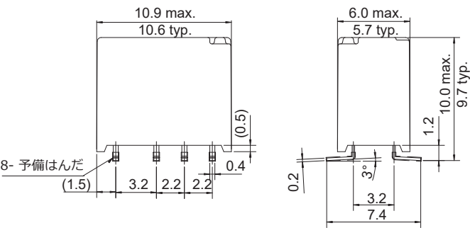
●外形寸法図
