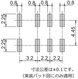
●実装パッド図 (TOP VIEW)
