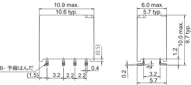
●外形寸法図
