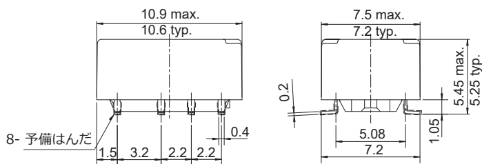
●外形寸法図
