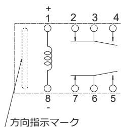
●端子配列・内部結線図 (BOTTOM VIEW)
