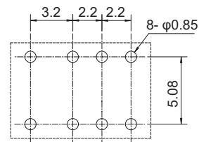
●基板孔開け図 (BOTTOM VIEW)
