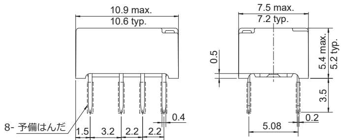
●外形寸法図
