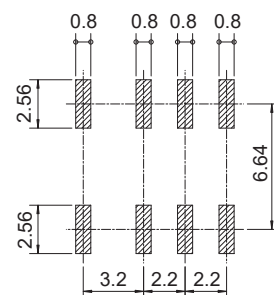
●実装パッド図 (TOP VIEW)
