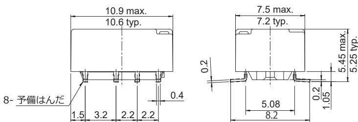
●外形寸法図
