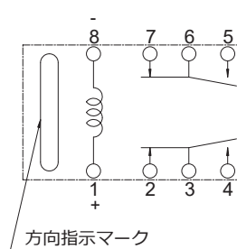
●端子配列・内部結線図 (TOP VIEW)
