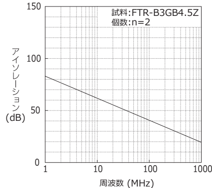
高周波特性
