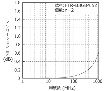
高周波特性
