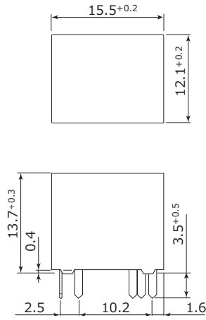
●外形寸法図
