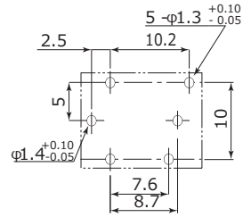
●基板孔開け図
